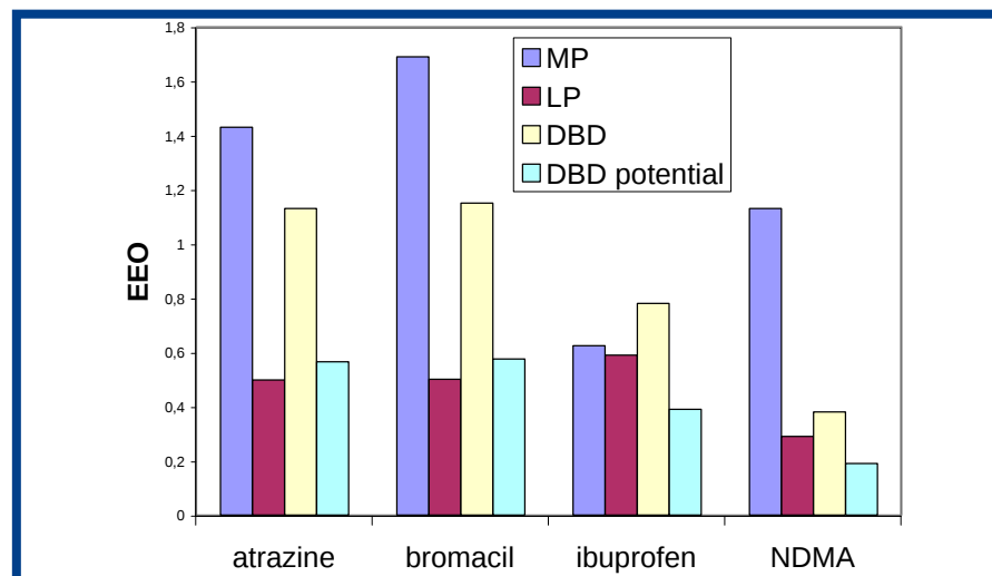
Afb. 1: E_{EO} -waarden bij Dunea voor verschillende pilotreactoren. MP = MD, LP = LD, potential = geoptimaliseerd.
